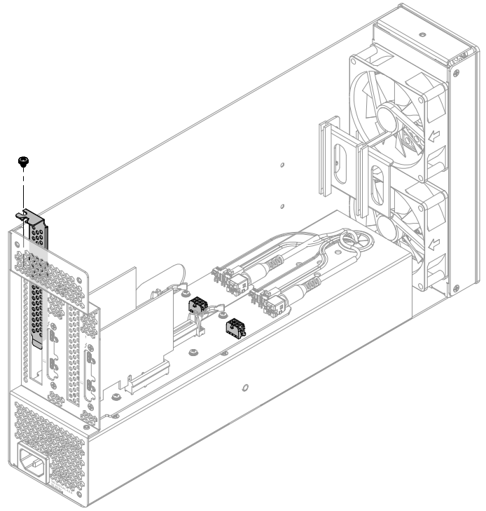
Step 2 / Étape 2
