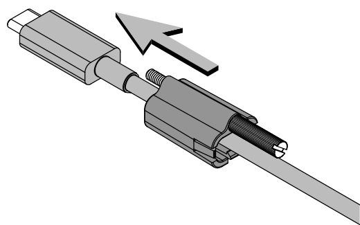
Step 5 / Étape 5
