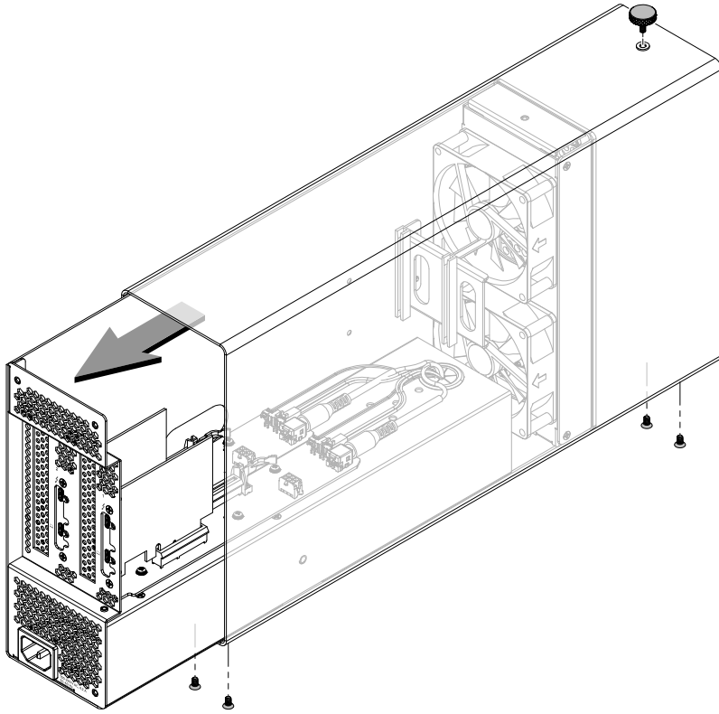
Step 1 / Étape 1
