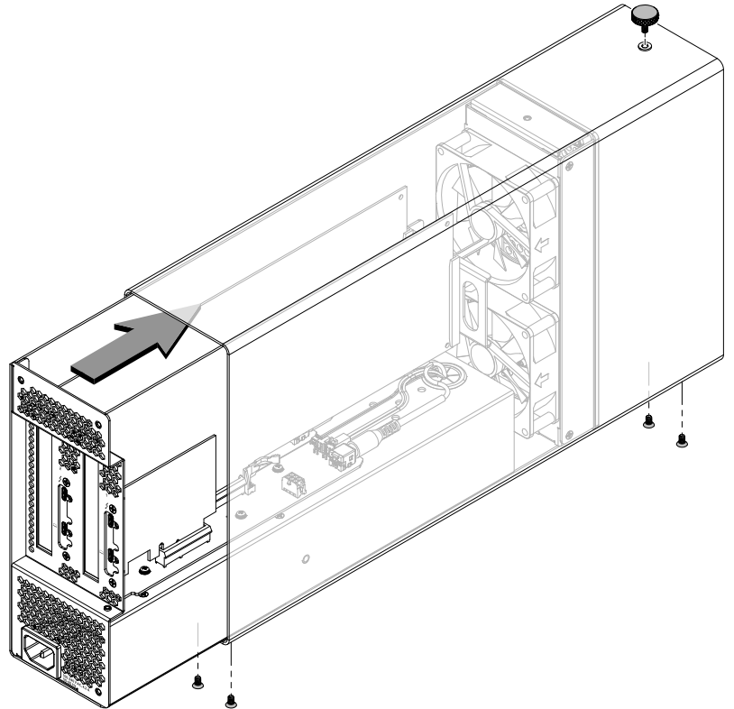
Step 4 / Étape 4
