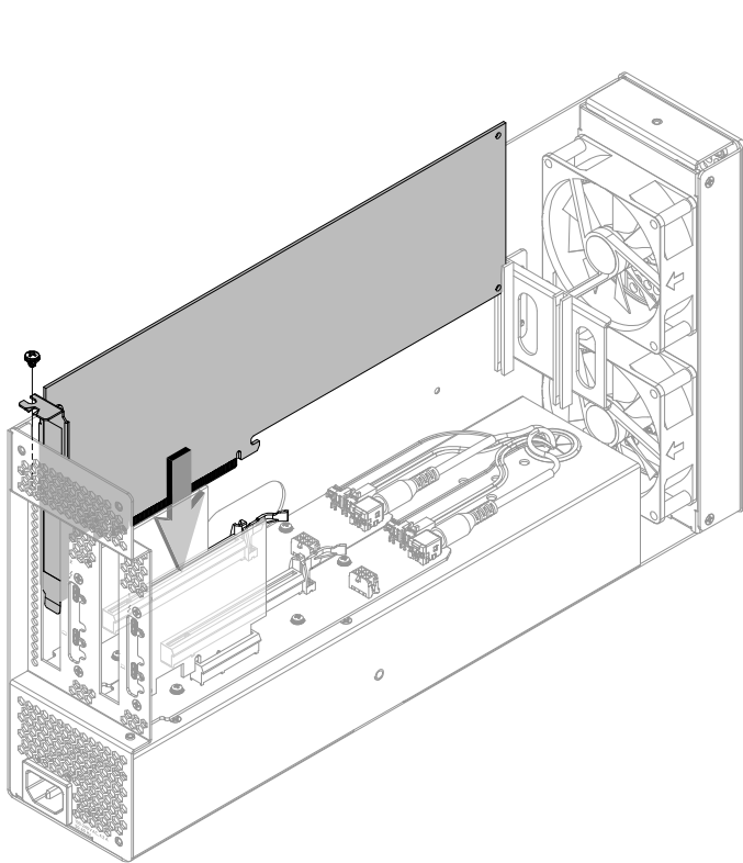
Step 3 / Étape 3
