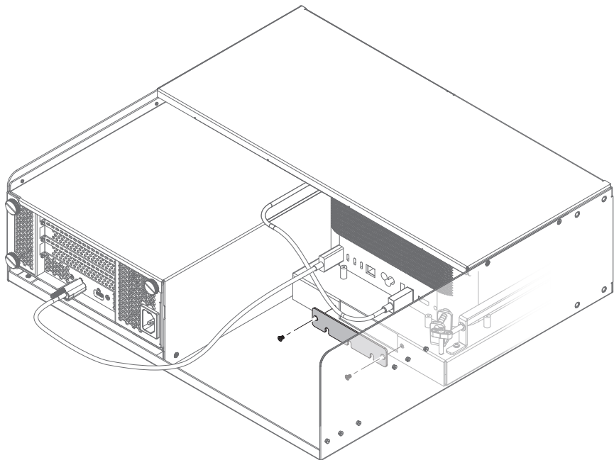
Step 8 / Étape 8
