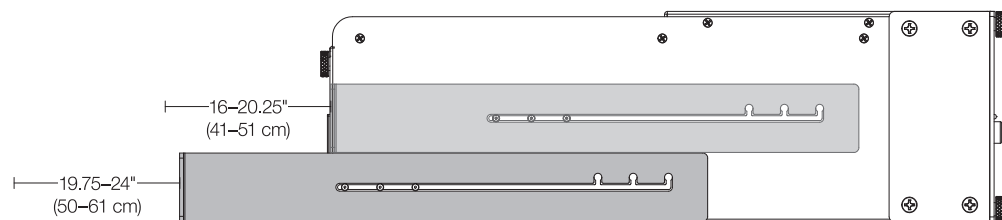
Step 14 / Étape 14
